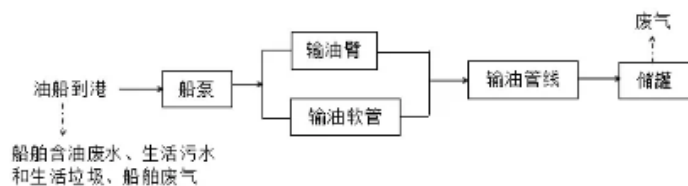
图4-1 油品卸船作业工艺流程示意图
