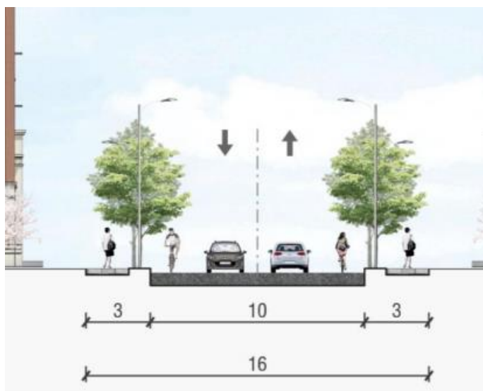
图2-3 纬一路横断面设计图
