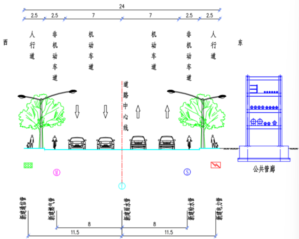
图2-6 兴盛路设计管位图
