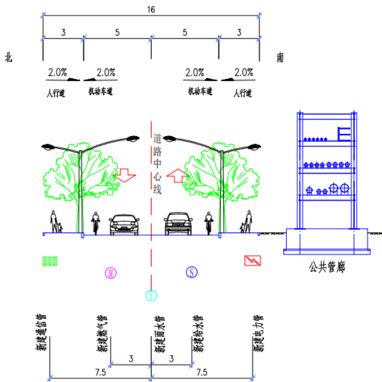
图2-8 纬一路设计管位图
