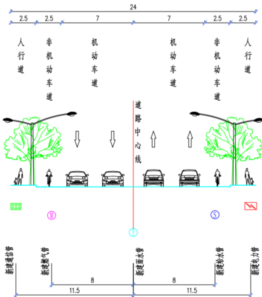
图2-5 滨海路设计管位图
