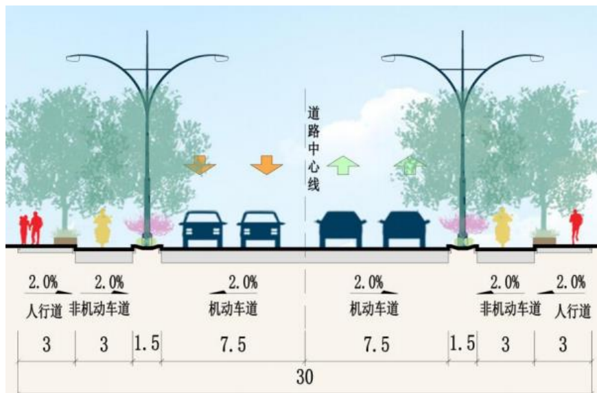
图2-1 工业路横断面设计图
