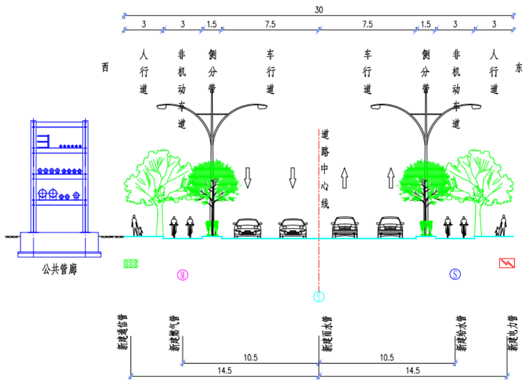
图2-7 工业路设计管位图
