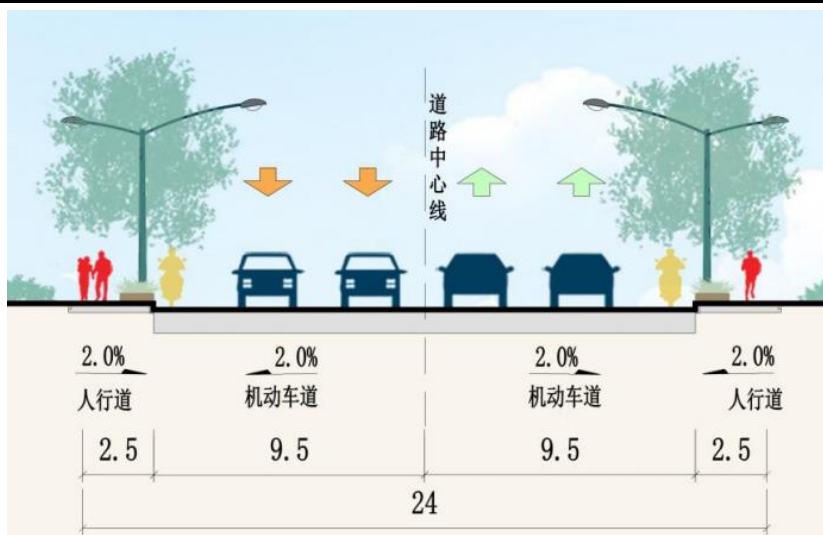
图2-2 兴盛路、滨海路横断面设计图
