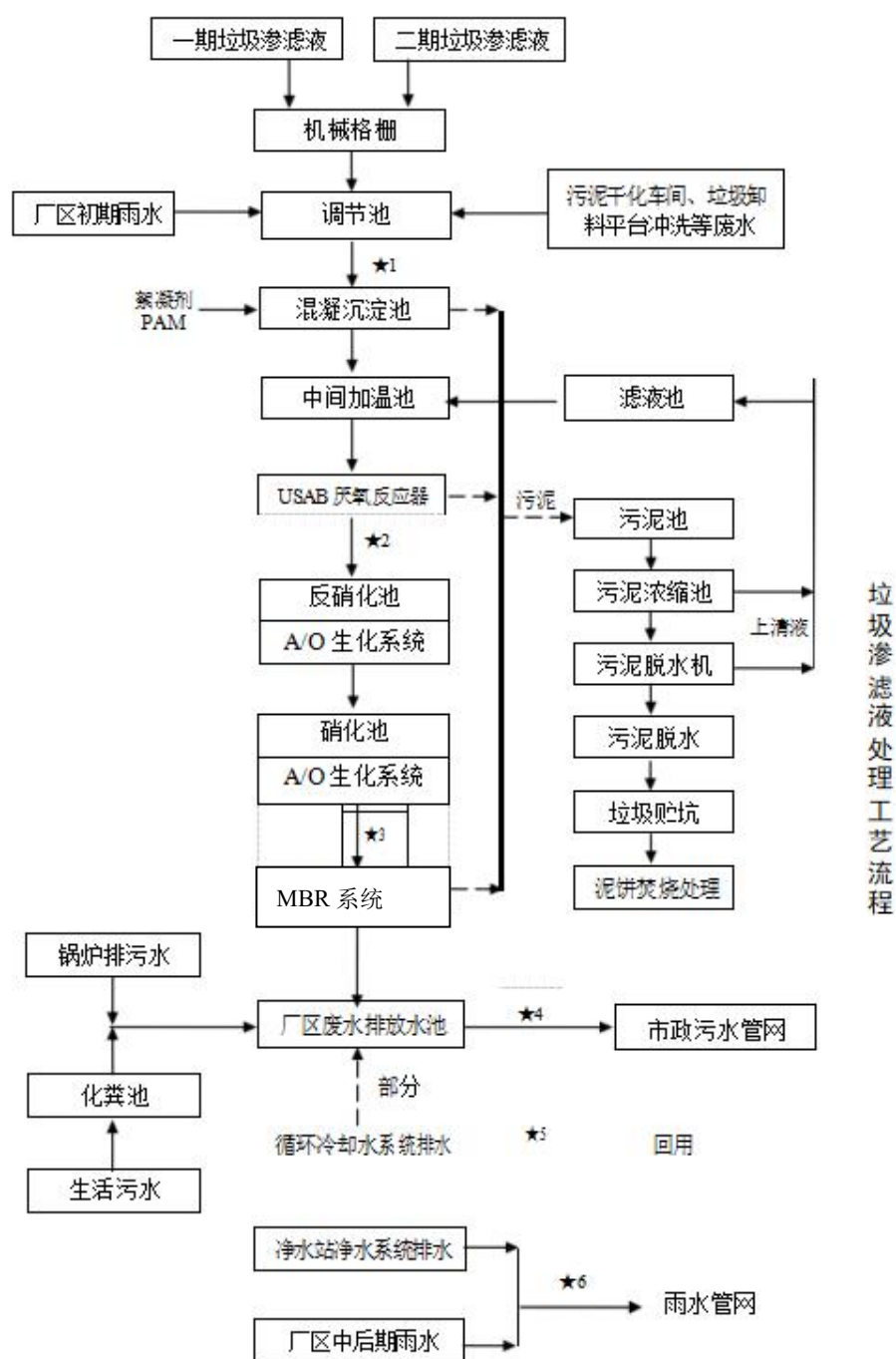
图 2-4 污水处理工艺流程图
