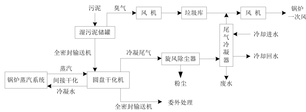
图 2-4 生产工艺流程（环评审批）
