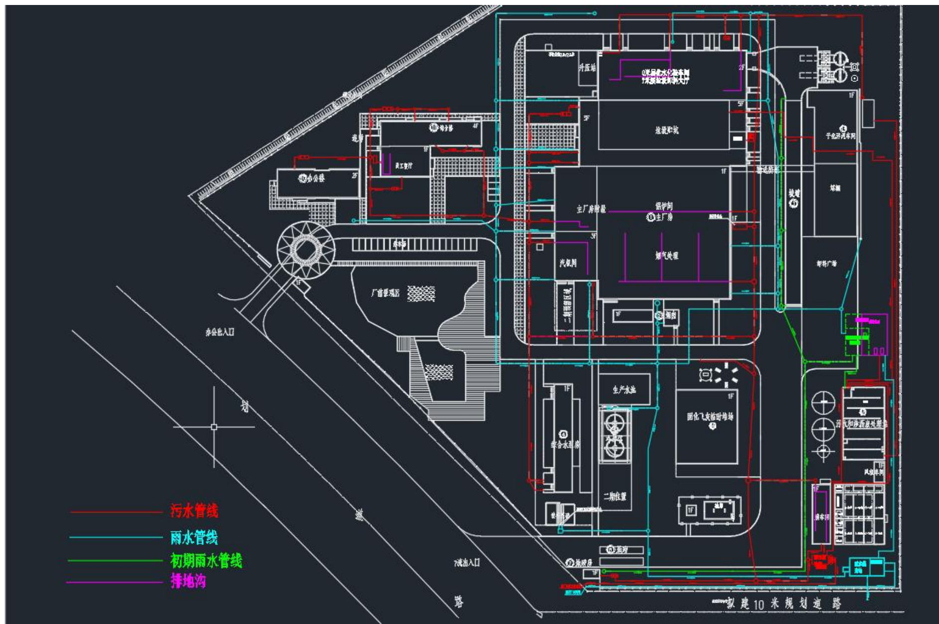
附图 4 企业雨污管网图
