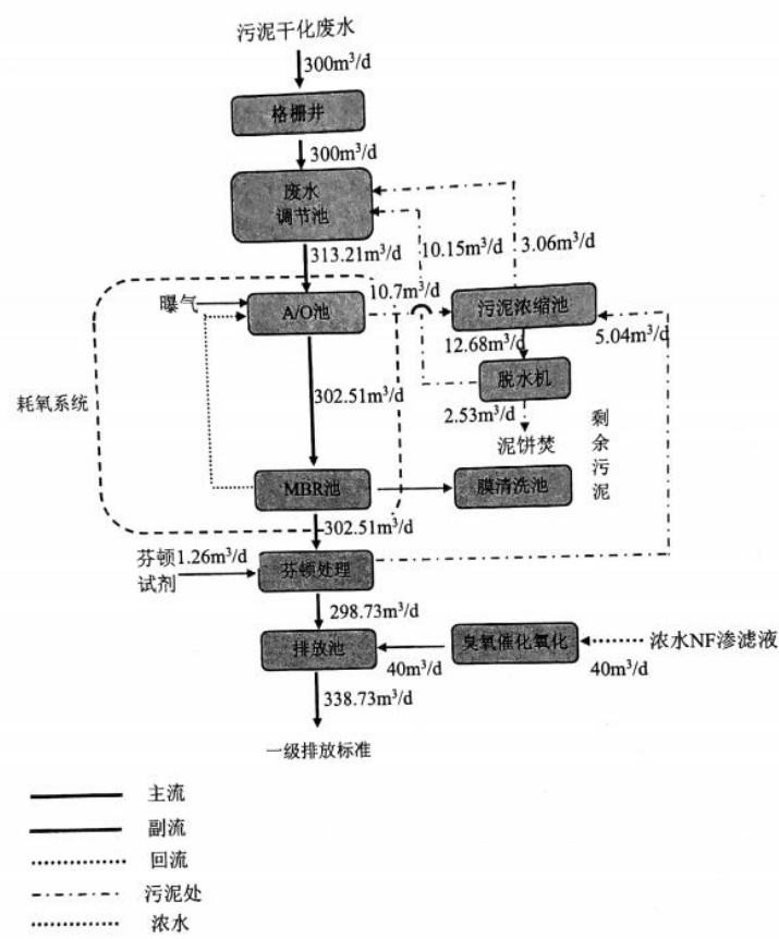
图 3-1 污泥干化废水处理工艺流程
