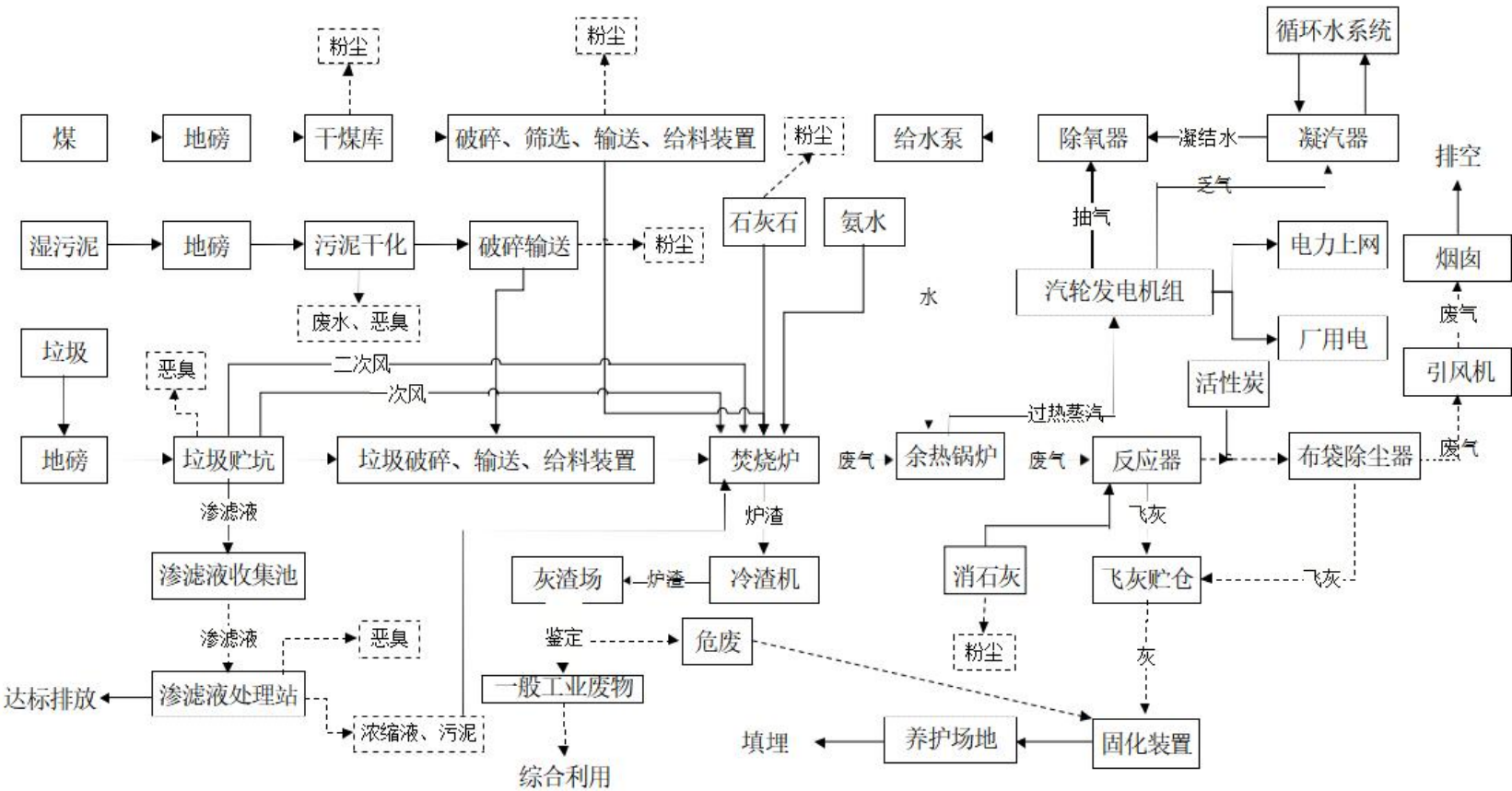
图 2-1 项目一期工艺流程图
